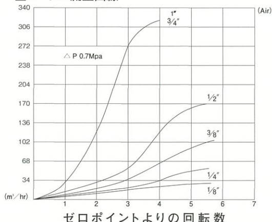
■ニードル流量曲線
