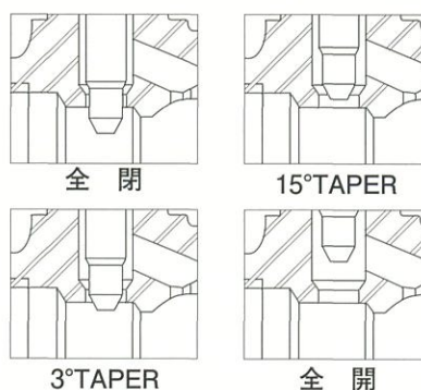
■スピンドル形状
