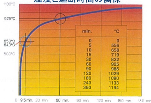
温度と遮断時間の関係
